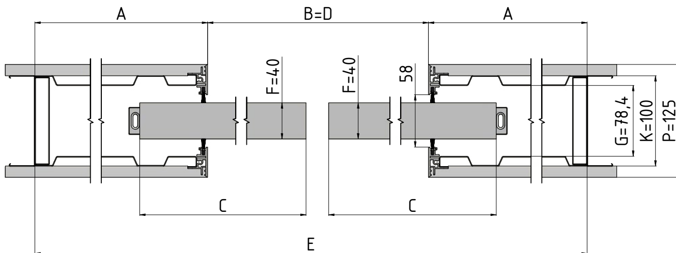
Horizontální řez pouzdra AKTIVE II KOMFORT s dřevěným dveřním křídlem tloušťky 40 mm
