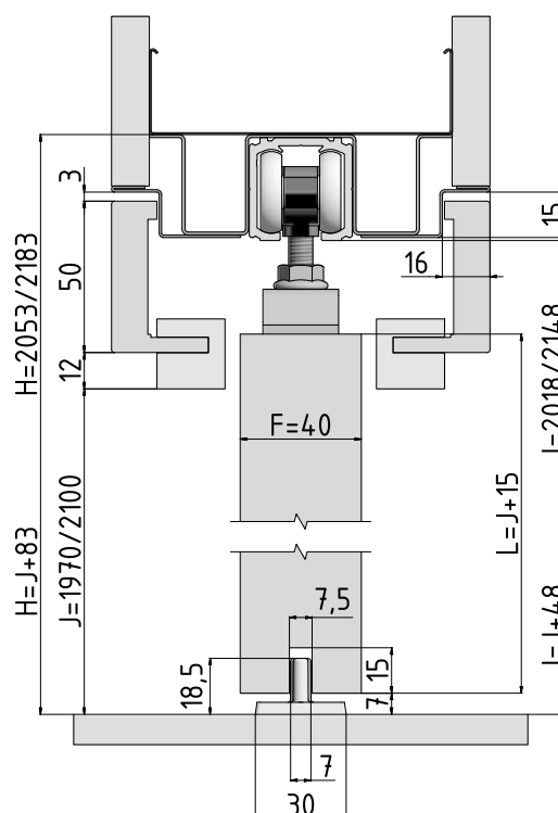
Vertikální řez pouzdra LATENTE KOMFORT s dřevěným dveřním křídlem tloušťky 40 mm
