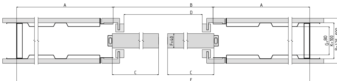
Horizontální řez pouzdra LATENTE KOMFORT s dřevěným dveřním křídlem tloušťky 40 mm
